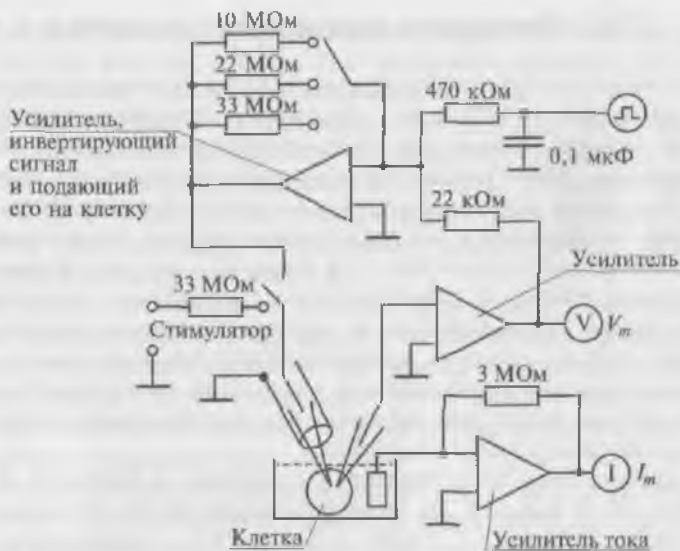
Рис. 7.8. Блок схема установки для исследования клеток (например, нервных) методом фиксации потенциала с двумя микроэлектродами. Точковый микроэлектрод экранирован
