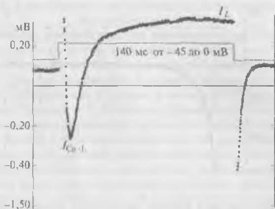
Рис. 11.11. Входящий Ca^{2+} -ток через L-тип Ca^{2+} -каналов ( I_{Ca-L} ) и выходящий K^+ -ток рабочего кардиомиоцита мыши, зарегистрированный методом patch-clamp в конфигурации whole-cell при смещении мембранного потенциала до 0 мВ относительно поддерживаемого потенциала величиной -45 мВ. Поздний ток, исследуемый при растяжении клетки, обозначен как I_T и определяется на последних 10 мс смещающего потенциала. Na^+ -ток подавлен поддерживаемым на уровне -45 мВ потенциалом
