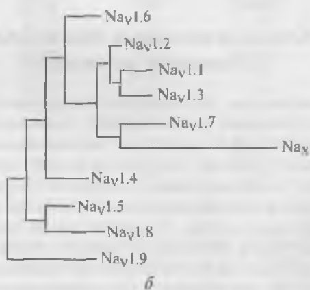
Рис. 8.4. Подобие последовательности аминокислот и филогенетические взаимоотношения \alpha -субъединиц потенциалуправляемых \text{Na}^+ -каналов:
