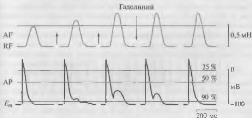
Рис. 11.40. Ингибирование гадолинием, добавленным в перфузионный раствор в концентрации 40 мкмоль/л; SID на уровне APD90:
