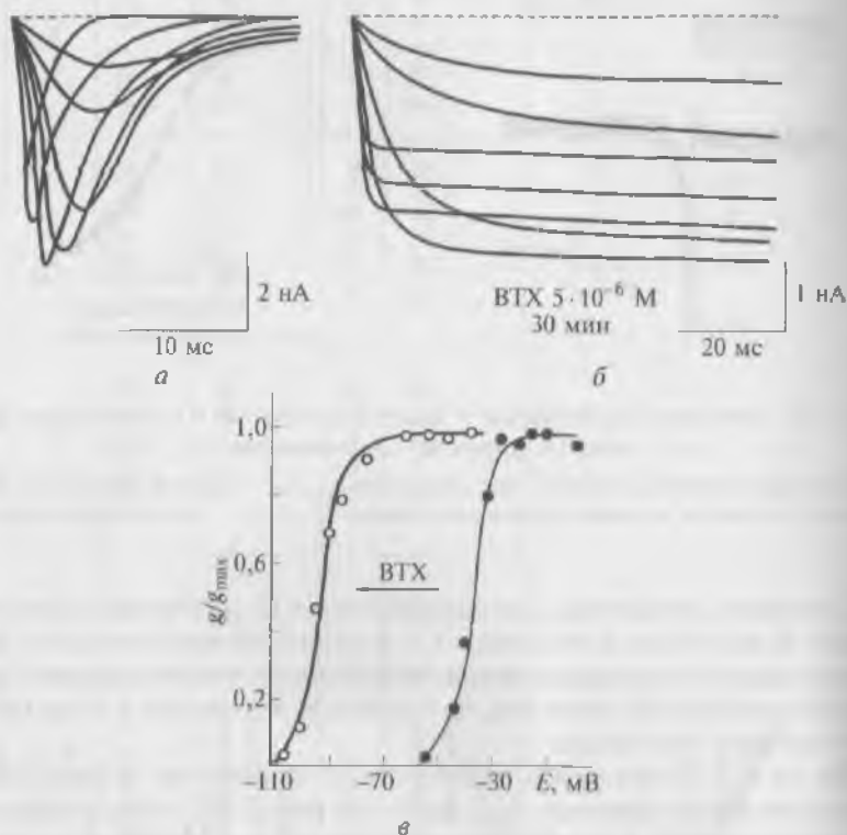
Рис. 7.31. Влияние батрахотоксина на Na^+ -токи нейробластомы:
