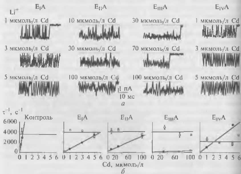
Рис. 9.13. Мутанты с единичным аланином в EEEE-локусе различаются между собой по кинетике \text{Cd}^{2+} -блока:
