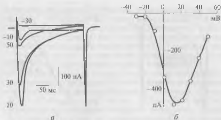
Рис. 9.18. Типичный whole-cell \text{Ca}^{2+} -ток ( I_{\text{Ca-L}} ), зарегистрированный от изолированного кардиомиоцита желудочков мышцы, мембрана которого имеет \text{Ca}_V1 -каналы:
