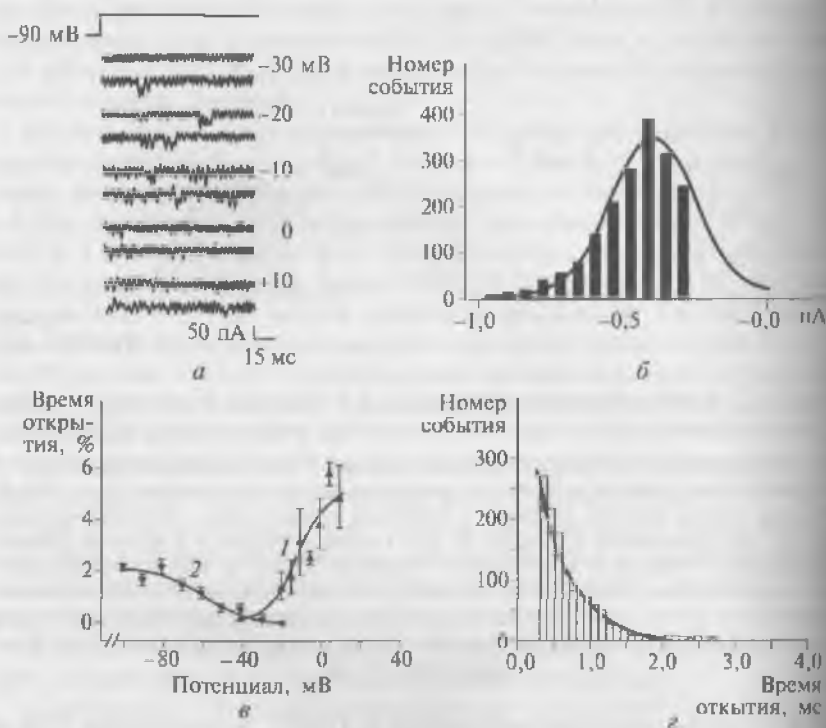
Рис. 9.23. Биофизические свойства канала подсемейства \text{Ca}_v3 на примере \text{Ca}_v3.2 -канала с Т-типом \text{Ca}^{2+} -тока, зарегистрированного в cell-attached patch у клеток НЕК-293:
