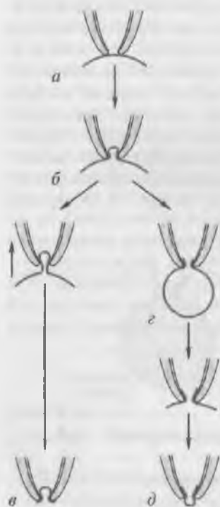
Рис. 7.12. Схема различных конфигураций patch-clamp (а—д)
