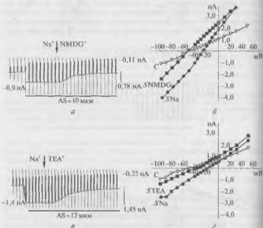
Рис. 11.50. Ток SAC может переноситься NMDG + и TEA + , однако с низкой проводимостью. K + -токи подавлены, раствор — Ca 2+ -free PSS. Клетки предварительно были диализованы раствором BAPTA (5 ммоль/л):
