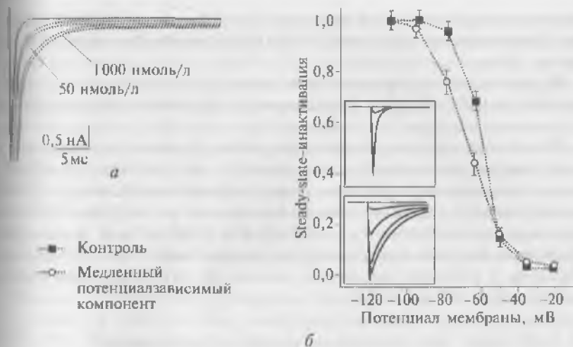
Рис. 8.36. Эффект одного из токсинов морских анемонов АТХ-II из Anemonia sulcata на ток через \text{Na}_v1.4 -каналы в культуре клеток НЕК-293 при смешении потенциала от -110 до -20 мВ:
