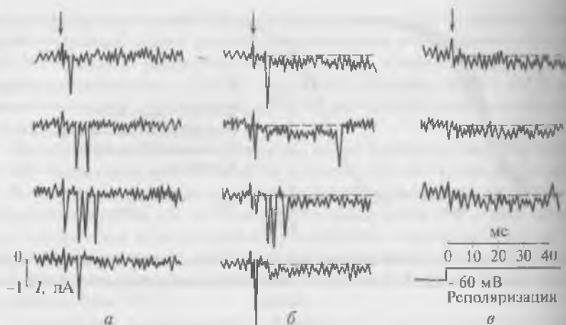
Рис. 8.27. Регистрация intactных и модифицированных вератридином одиночных \text{Na}^+ -каналов в клетке нейробластомы на фоне деполяризации клетки до -60 мВ:
