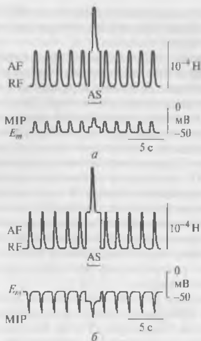
Рис. 11.70. Синхронная регистрация механограммы предсердия (верхняя кривая) и механоиндуцированных потенциалов фибробластов (нижняя кривая):
