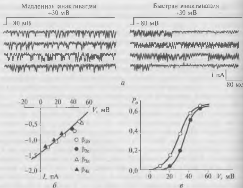
Рис. 9.20. Биофизические свойства \text{Ca}_v2.1 -канала с P/Q-типом \text{Ca}^{2+} -тока, зарегистрированного в cell-attached patch у клеток HEK-293:
