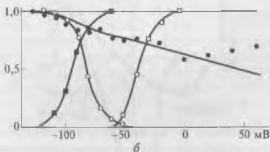
Рис. 8.23. Модификация аконитином \text{Na}^+ -каналов:
