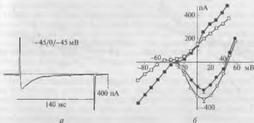
Рис. 11.35. Пример L-типа \text{Ca}^{2+} -тока ( I_{\text{Ca-L}} ) и позднего тока ( I_L ), измеренного в конце деполяризующего импульса длительностью 140 мс у предсердного кардиомиоцита человека на фоне ингибирования \text{K}^+ -тока ( I_{\text{K1}} ):
