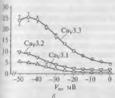
Рис. 9.24. Типичные оригинальные кривые \text{Ca}^{2+} -тока, зарегистрированные от \text{Ca}_v3.1 -, \text{Ca}_v3.2 - и \text{Ca}_v3.3 -каналов в конфигурации whole-cell: a — \text{Ca}^{2+} -токи зарегистрированы на фоне ступенек деполяризации до -45 мВ от поддерживаемого потенциала величиной -90 мВ; b — активационные кривые для трех типов каналов; v — инактивационные кривые для этих же каналов
