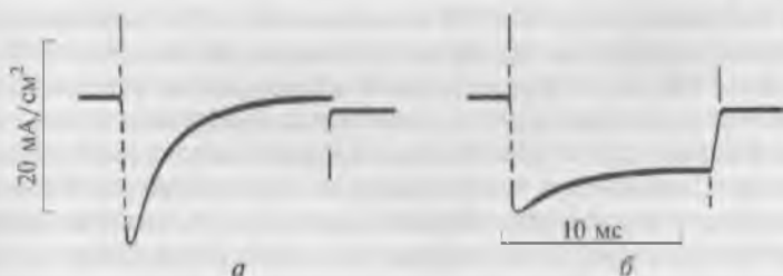
Рис. 8.29. Влияние яда скорпиона ( Leiurus quinquestriatus ) на \text{Na}^+ -ток перехвата Ранвье:
