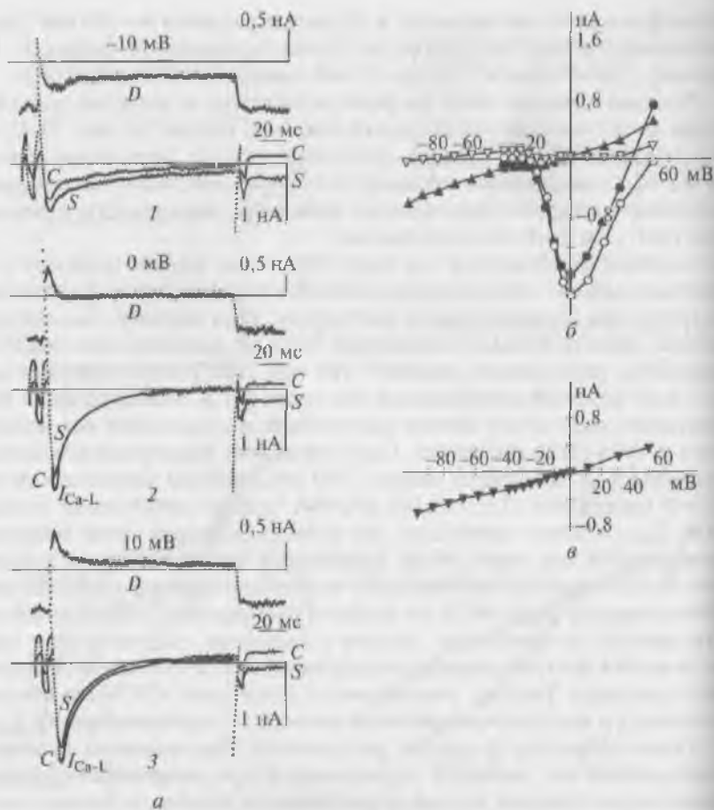
Рис. 11.46. Активация растяжением неселективного катионного тока при растяжении кардиомиоцита желудочка морской свинки на 8 мкм в условиях подавленного цезием калиевого тока:
