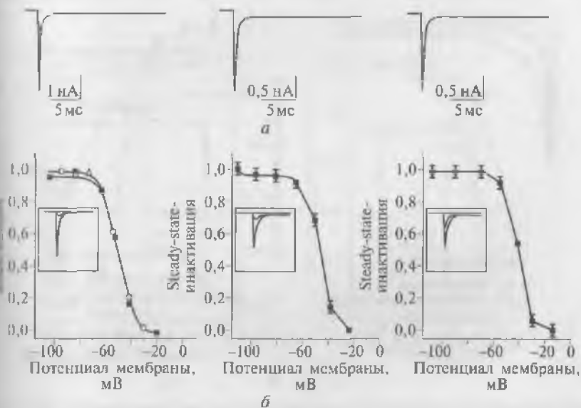
Рис. 8.32. Входящий ток через Na_v1.1 -каналы:
