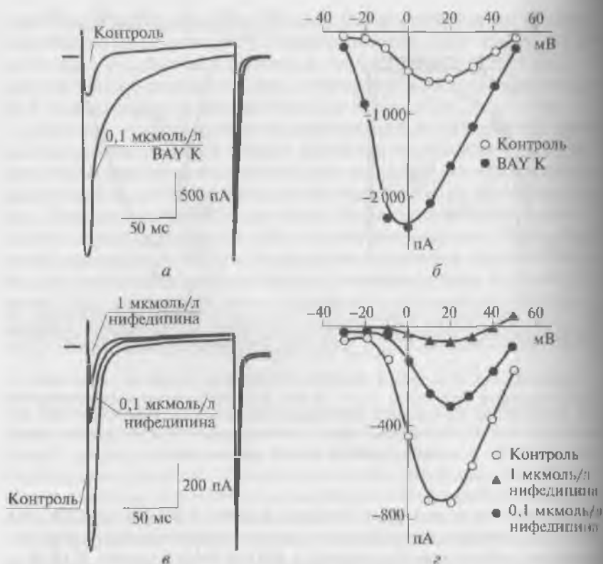
Рис. 9.19. Примеры действия фармакологических препаратов на типичный whole-cell Ca^{2+} -ток ( I_{Ca-L} ), зарегистрированный от изолированного кардиомиоцита желудочков мыши, мембрана которого имеет Ca_v1 -каналы:
