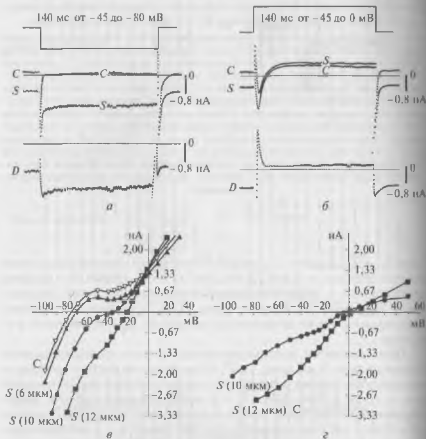
Рис. 11.45. Модуляция базового мембранного тока под действием растяжения на 8 мкм изолированного кардиомиоцита желудочка морской свинки. К + -ток не подавлен, т.е. и в перфузионном растворе, и в пипетке находятся К + -катионы:
