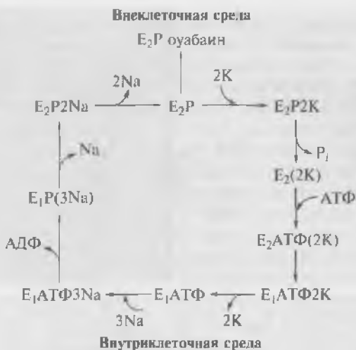
Рис. 3.14. Схема механизма переноса ионов Na^+ и K^+ с помощью Na^+/K^+ -АТФазы
