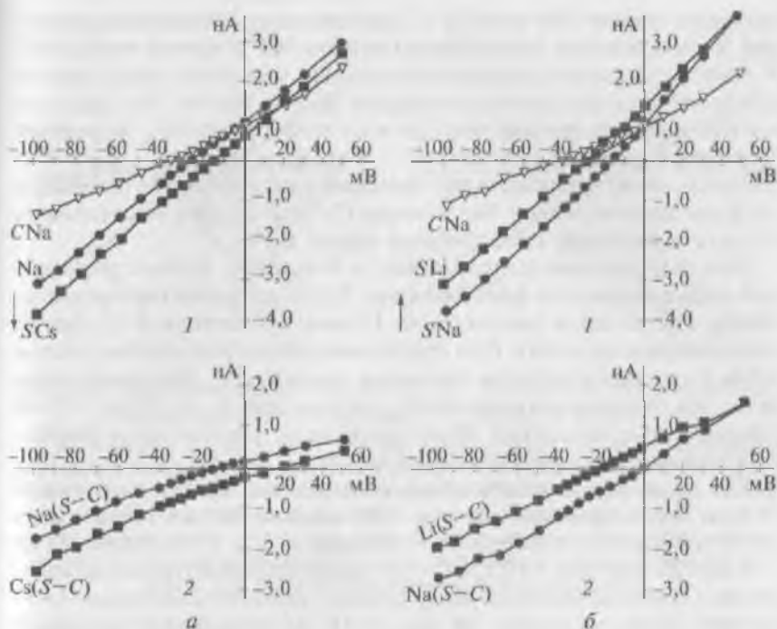
Рис. 11.51. Токи SAC могут переноситься ионами Cs^+ или Li^+ . K^+ -токи подавлены. Раствор — Ca^{2+} -free PSS. Клетки предварительно были диализованы раствором ВАРТА (5 ммоль/л):
