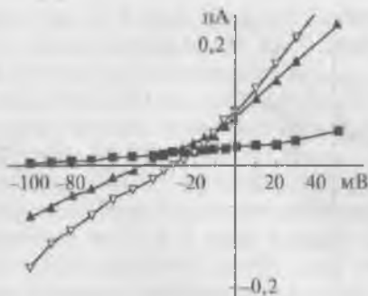
Рис. 11.84. Растяжение клетки меняет базовую мембранную проводимость. Точка пересечения I-V -кривой для I_L с осью потенциала является потенциалом ( E_0 ) при токе, равном нулю. Контрольная кривая I_L (пустые треугольники, E_0 = -28 мВ), кривая I_L при растяжении клетки на 2 мкм (заполненные треугольники, E_0 = -45 мВ), кривая I_L через 5 мин после добавления 8 мкмоль/л Gd^{3+} на фоне продолжающегося растяжения фибробласта (заполненные квадраты, E_0 = -110 мВ)
