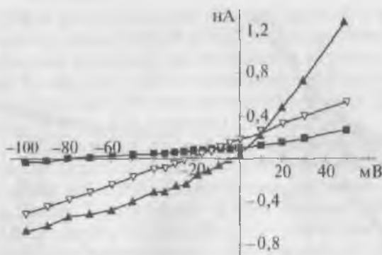
Рис. 11.80. Сжатие клетки увеличивает базовую мембранную проводимость. Точка пересечения I-V -кривой для I_L с осью потенциала является потенциалом ( E_0 ) при токе, равном нулю. Контрольная кривая I_L (пустые треугольники, E_0 = -25 мВ), кривая I_L при сжатии клетки на 3 мкм (заполненные треугольники, E_0 = -5 мВ), кривая I_L через 5 мин после добавления 8 мкмоль/л Gd^{3+} на фоне продолжающегося сжатия фибробласта (заполненные квадратики, E_0 = -90 мВ)
