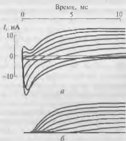
Рис. 8.14. Типичное блокирующее действие тетродотоксина на \text{Na}^+ -ток: a — контроль: суммарный ток, включающий входящий \text{Na}^+ -ток и выходящий ток, возникающий при разных степенях деполяризации относительно поддерживаемого потенциала; б — полное ингибирование входящего \text{Na}^+ -тока тетродотоксином в концентрации 300 нмоль/л
