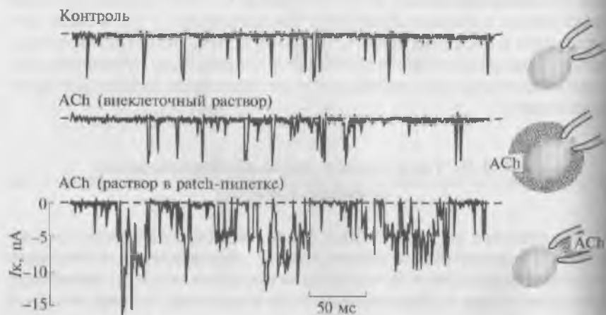
Рис. 4.18. Регистрация входящего \text{K}^+ -тока, протекающего через \text{K}^+ -канал, активируемый \text{ACh} , — \text{K}(\text{ACh}) -канал, в cell-attached конфигурации. Верхняя кривая демонстрирует контрольную регистрацию, средняя кривая показывает регистрацию на фоне введенного в перфузионный раствор \text{ACh} в концентрации 100 \text{ нмоль/л} . Нижняя кривая демонстрирует регистрацию на фоне введенного в patch-пипетку \text{ACh} в концентрации 10 \text{ нмоль/л}
