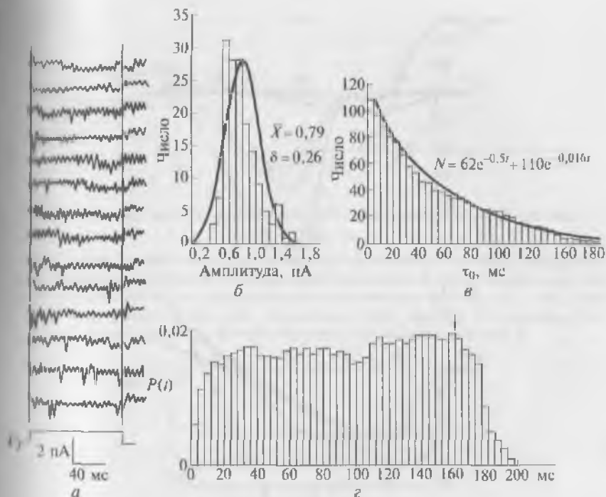
Рис. 8.20. Влияние ВТХ на Na + -канал нейробластомы и его основной анализ:
