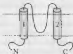
Рис. 10.4. Молекулярная организация K^+ -каналов с максимальным выпрямления с током входящего направления ( K_{ir} )
