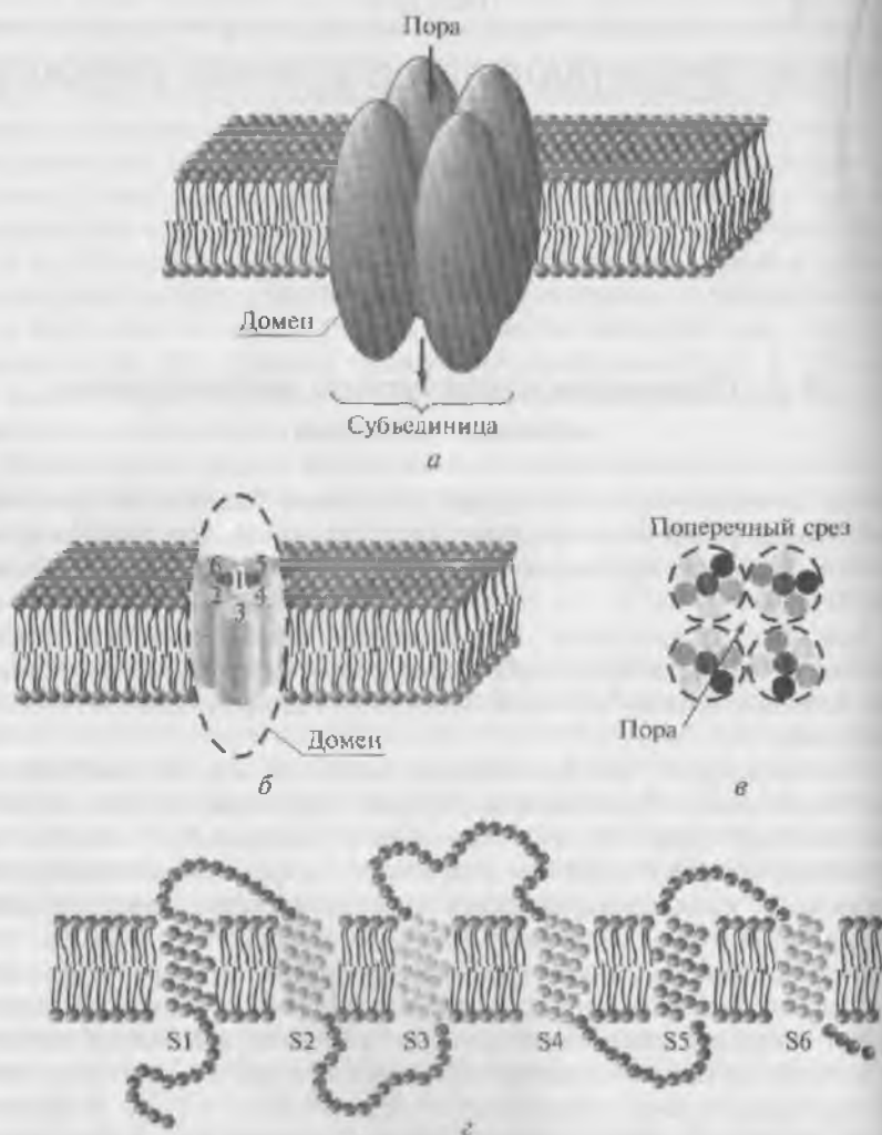
Рис. 4.1. Принципиальная модель молекулярной организации ионного канала на основе порообразующей мембранной \alpha -субъединицы, состоящей из четырех доменов:
