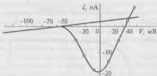
Рис. 7.21. Вольт-амперные характеристики, построенные по пиковым (кружки) и стационарным значениям токов, продемонстрированных на рис. 7.20
