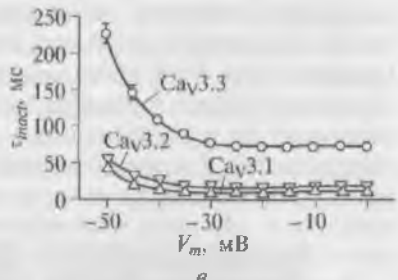
Рис. 9.24. Типичные оригинальные кривые \text{Ca}^{2+} -тока, зарегистрированные от \text{Ca}_v3.1 -, \text{Ca}_v3.2 - и \text{Ca}_v3.3 -каналов в конфигурации whole-cell: a — \text{Ca}^{2+} -токи зарегистрированы на фоне ступенек деполяризации до -45 мВ от поддерживаемого потенциала величиной -90 мВ; b — активационные кривые для трех типов каналов; v — инактивационные кривые для этих же каналов
