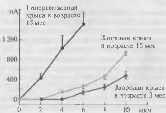
Рис. 11.64. Зависимость величины I_{SAC} от величины растяжения клетки. Показаны кардиомиоциты желудочка сердца здоровой крысы (3 мес и 15 мес) и гипертонической крысы (15 мес)
