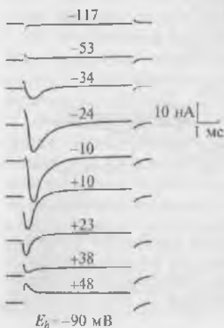
Рис. 7.20. \text{Na}^+ -токи, зарегистрированные методом patch-clamp в конфигурации whole-cell. Величина поддерживаемого потенциала E_h равна -90 мВ. Величины ступенек тестирующих потенциалов указаны на рисунке
