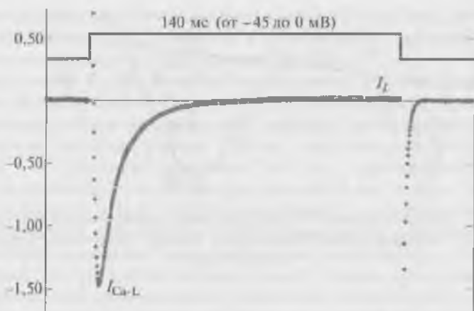
Рис. 7.22. Ca^{2+} -ток вентрикулярного кардиомиоцита, зарегистрированный методом patch-clamp в конфигурации whole-cell, при смещении мембранного потенциала до 0 мВ относительно поддерживаемого потенциала величиной -45 мВ. Na^+ -ток подавлен поддерживаемым на уровне -45 мВ потенциалом, а K^+ -ток подавлен ионами Cs^+ , являющимися блокаторами K^+ -каналов. На рисунке представлен также поздний ток ( I_L ), сохраняющийся после блокады K^+ -тока ионами Cs^+
