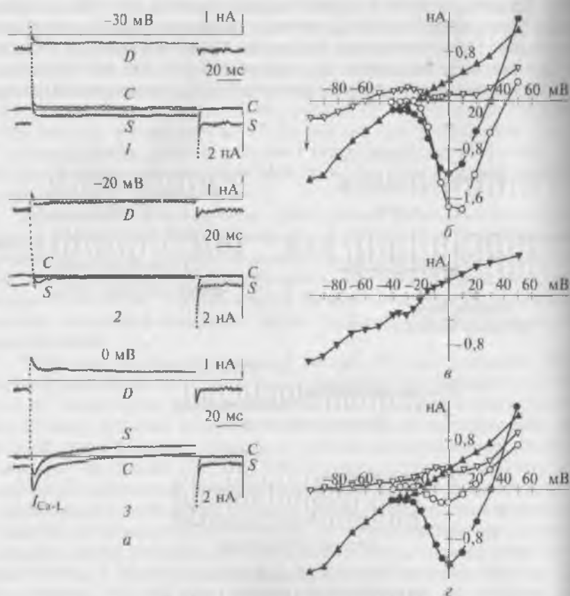
Рис. 11.63. Активация растяжением на 4 \mu м Gd^{3+} -сенситивного неселективного катионного тока при растяжении кардиомиоцита левого желудочка человека после инфаркта миокарда в условиях подавленного цезием калиевого тока:
