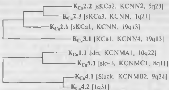
Рис. 10.3. Филогенетическое дерево для K_{Ca} -каналов. Первая группа включает в себя K_{Ca}2 , K_{Ca}3 -каналы, вторая — K_{Ca}1 -, K_{Ca}4 -, K_{Ca}5 -каналы. Новые каналы пока еще не были добавлены к этой топологии
