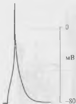
Рис. 7.16. Потенциал действия у изолированного вентрикулярного кардиомиоцита мышцы, зарегистрированный методом patch-clamp в режиме current clamp в конфигурации whole-cell
