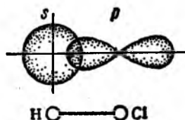
Рис. 9. Линейная форма молекулы \text{HCl}
