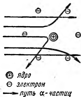
Рис. 3. Рассеяние \alpha -частиц, приближающихся к атомному ядру
