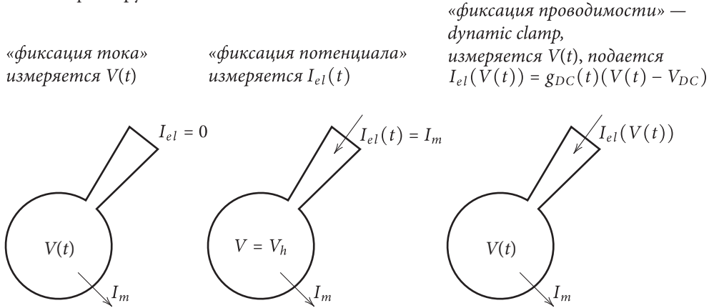
Рис. 4. Режимы фиксации тока, фиксации потенциала и dynamic clamp при измерениях patch-электродом в режиме whole-cell .
