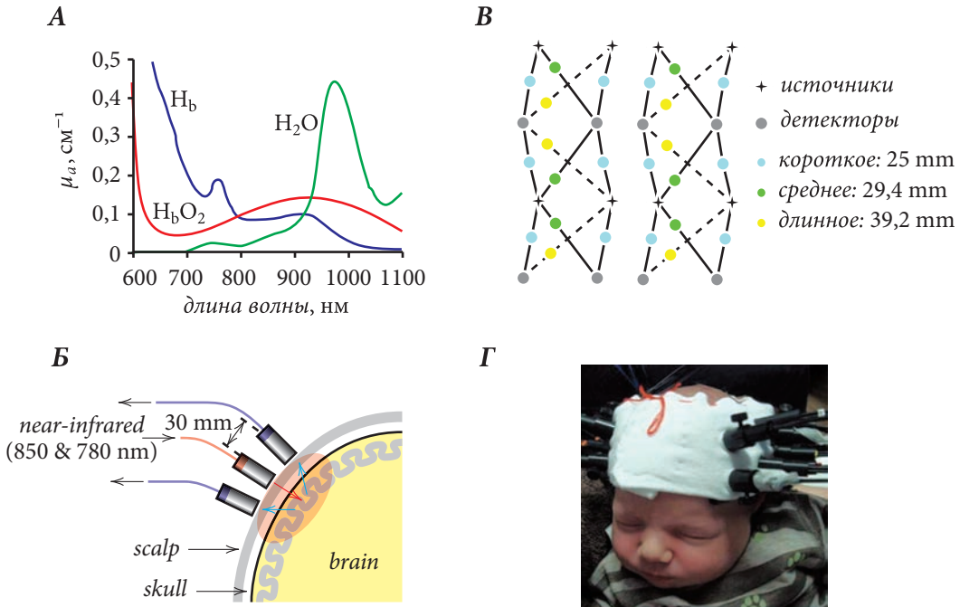
Рис. 5. А) Зависимость коэффициента поглощения дезокси-гемоглобина (H b ), оксигемоглобина (H b O 2 ) и воды (H 2 O) в зависимости от длины. Б) Падение интенсивности монохромного света, излучаемого лазерным диодом и проходящего через поверхностные слои скальпа, мозговых оболочек и коры мозга, но не проникающего глубже нескольких сантиметров, регистрируется с наибольшей вероятностью на поверхности головы на расстоянии нескольких см от источника — траектория распространения света от источника до детектора таким образом имеет банановидную форму. В) Расположение NIRS сенсоров-каналов, образованных парами источников и детекторов монохромного света. Г) В нашем исследовании на новорожденных, мы использовали систему для измерения гемодинамического ответа методом оптической спектроскопии около-инфракрасного излучения NIRS (Medical Physics Department, UCL, Великобритания), длины волн 780 and 850 нм.
