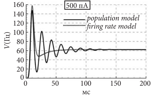
Рис. 11. Популяционная активность, вычисленная с помощью подробной популяционной модели (сплошная линия) и с помощью частотной модели (пунктир), основанной на ур. (9.2, 9.4–9.6). Нейроны популяции с момента t = 0 стимулировались постоянным током.
