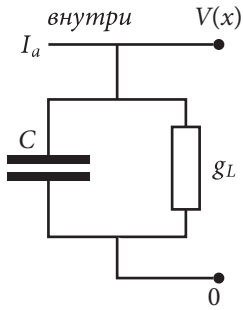
Рис. 2. Электрическая схема модели нейрона-порогового интегратора.
