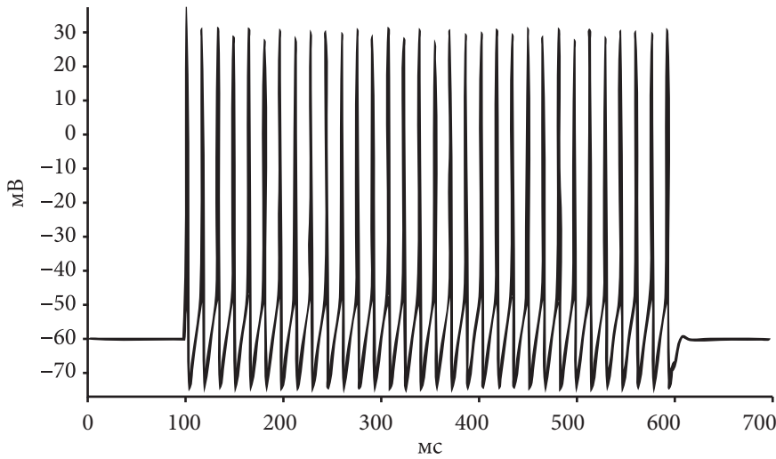
Рис. 6. Численное решение уравнений Ходжкина-Хаксли при задании стимулирующего тока I_{el} = 11 \mu\text{A}/\text{cm}^2 в период с 100 по 600 ms.
